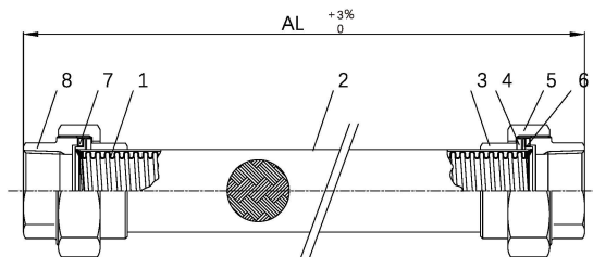
1.波纹管 2.软管 3.外环 4.内环 5.内接头 6.垫片 7.密封垫 8.外接头
